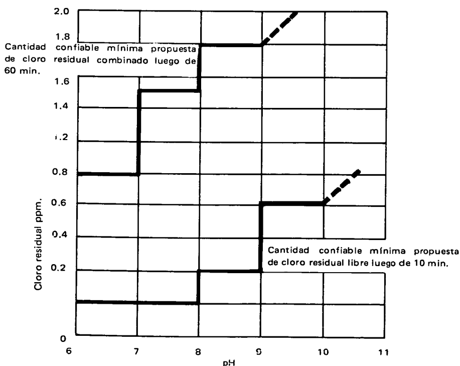
Figura 7-1 Cantidades mínimas de cloro residual disponible libre o combinado propuestas por Butterfield. (Fuente: Anónimo, 1951.)
