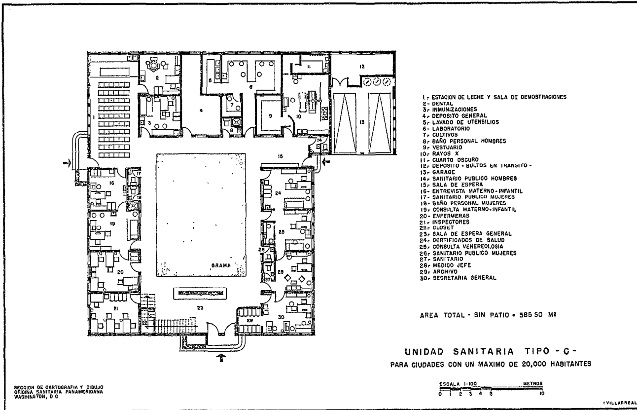
PLANO DE UNIDAD SANITARIA TIPO C ELABORADO POR EL MINISTERIO DE SANIDAD Y ASISTENCIA SOCIAL DE VENEZUELA
